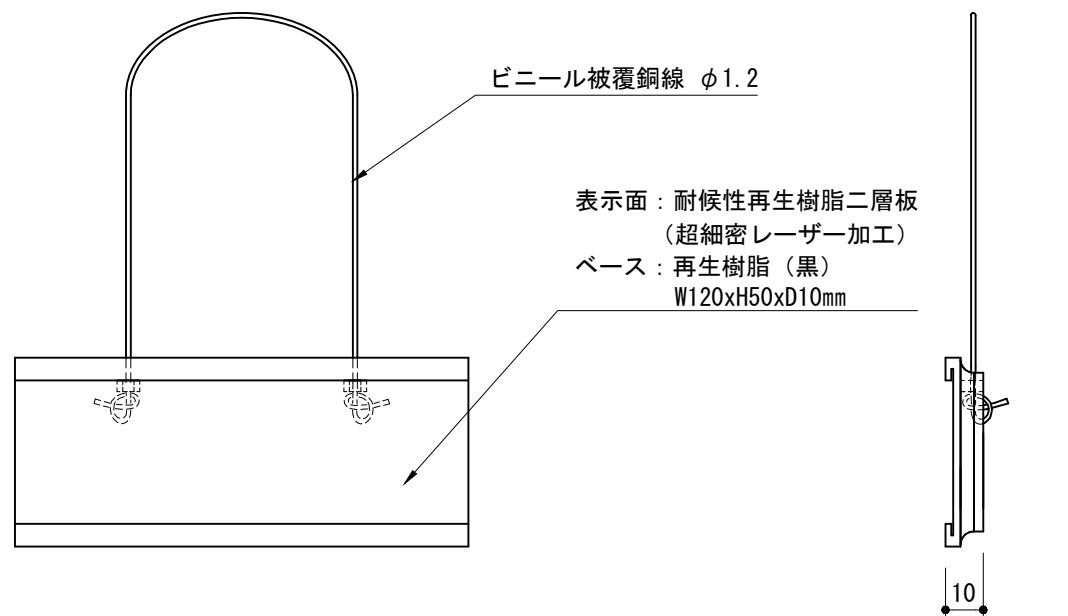
正面図 S=1:2
