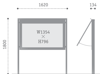
AGS-1618 本体サイズ：W1620×H1800×D134 表示板サイズ：W1354×H796
