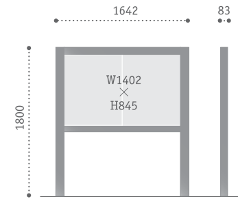
AGSP-1618 本体サイズ：W1642×H1800×D83 表示板サイズ：W1402×H845
