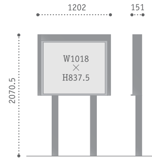
AGSL-1220 本体サイズ：W1202×H2070.5×D151 表示板サイズ：W1018×H837.5
