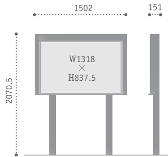
AGSL-1520 本体サイズ：W1502×H2070.5×D151 表示板サイズ：W1318×H837.5
