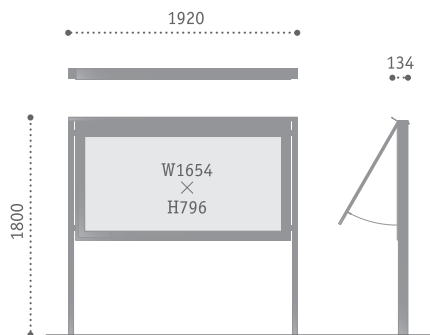
AGS-1918 本体サイズ：W1920×H1800×D134 表示板サイズ：W1654×H796
