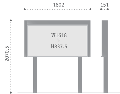
AGSL-1820 本体サイズ：W1802×H2070.5×D151 表示板サイズ：W1618×H837.5
