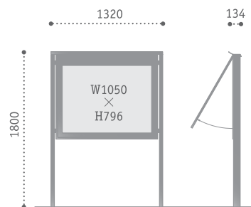
AGS-1318 本体サイズ：W1320×H1800×D134 表示板サイズ：W1050×H796
