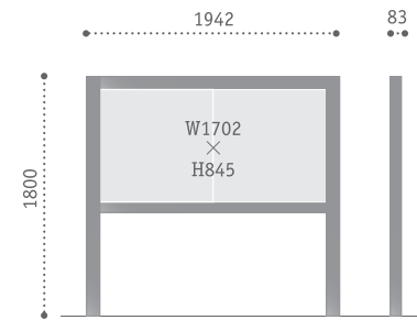
AGSP-1918 本体サイズ：W1942×H1800×D83 表示板サイズ：W1702×H845
