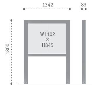
AGSP-1318 本体サイズ：W1342×H1800×D83 表示板サイズ：W1102×H845
