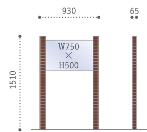
NL-915 本体サイズ：W930×H1510×D65 表示板サイズ：W750×H500
