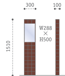
L-315 本 体サイズ：W300×H1510×D100 表示板サイズ：W288×H500
