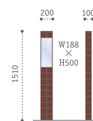
L-215 本 体サイズ：W200×H1510×D100 表示板サイズ：W188×H500
