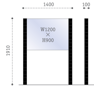
L-1419 本 体サイズ：W1400×H1910×D100 表示板サイズ：W1200×H900
