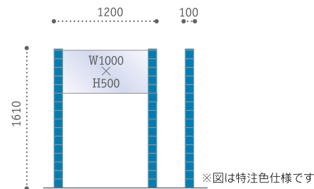
L-1216 本 体サイズ：W1200×H1610×D100 表示板サイズ：W1000×H500
