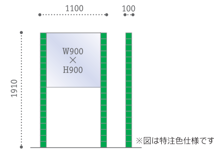
L-1119 本 体サイズ：W1100×H1910×D100 表示板サイズ：W900×H900
