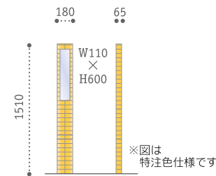
NL-115 本体サイズ：W180×H1510×D65 表示板サイズ：W110×H600
