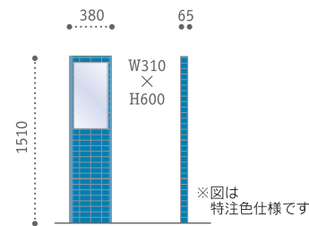
NL-315 本体サイズ：W380×H1510×D65 表示板サイズ：W310×H600
