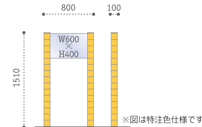
L-815 本 体サイズ：W800×H1510×D100 表示板サイズ：W600×H400
