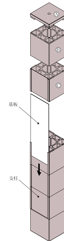
L-215 本 体サイズ：W200×H1510×D100 表示板サイズ：W188×H500
