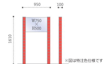
L-916 本 体サイズ：W950×H1610×D100 表示板サイズ：W750×H500
