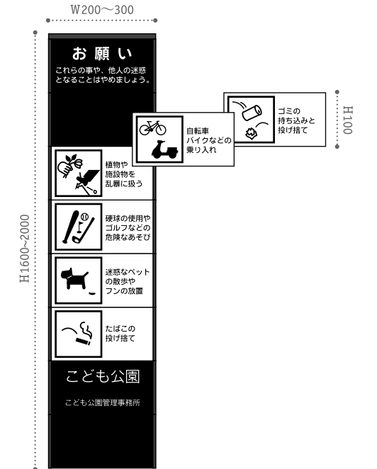
本体サイズ：W 200～300×H 1600～2000 表示方法：スーパーカラー「R」
