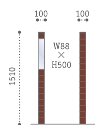
L-115 本 体サイズ：W100×H1510×D100 表示板サイズ：W88×H500
