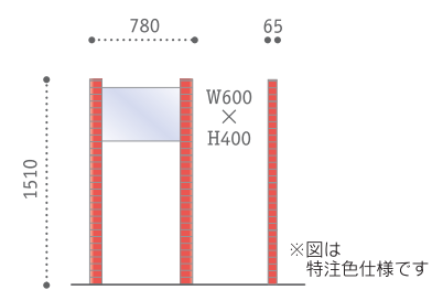
NL-715 本体サイズ：W780×H1510×D65 表示板サイズ：W600×H400
