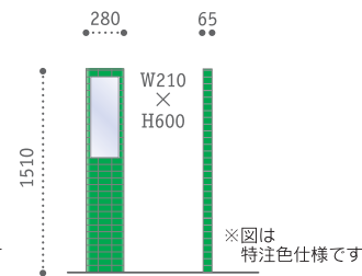
NL-215 本体サイズ：W280×H1510×D65 表示板サイズ：W210×H600
