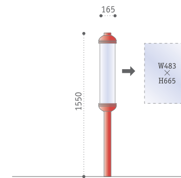
Y-115 本体サイズ：W165×H1550×D165 表示板サイズ：W483×H665
