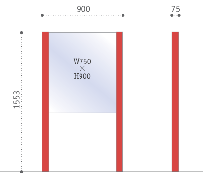
Y-915S 本体サイズ：W900×H1553×D75 表示板サイズ：W750×H900
