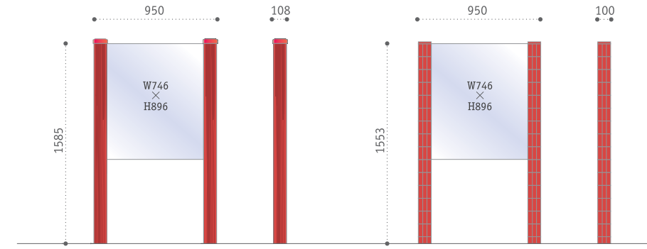
Y-915W 推奨品(イペ材) 本体サイズ：W950×H1585×D108 表示板サイズ：W746×H896
