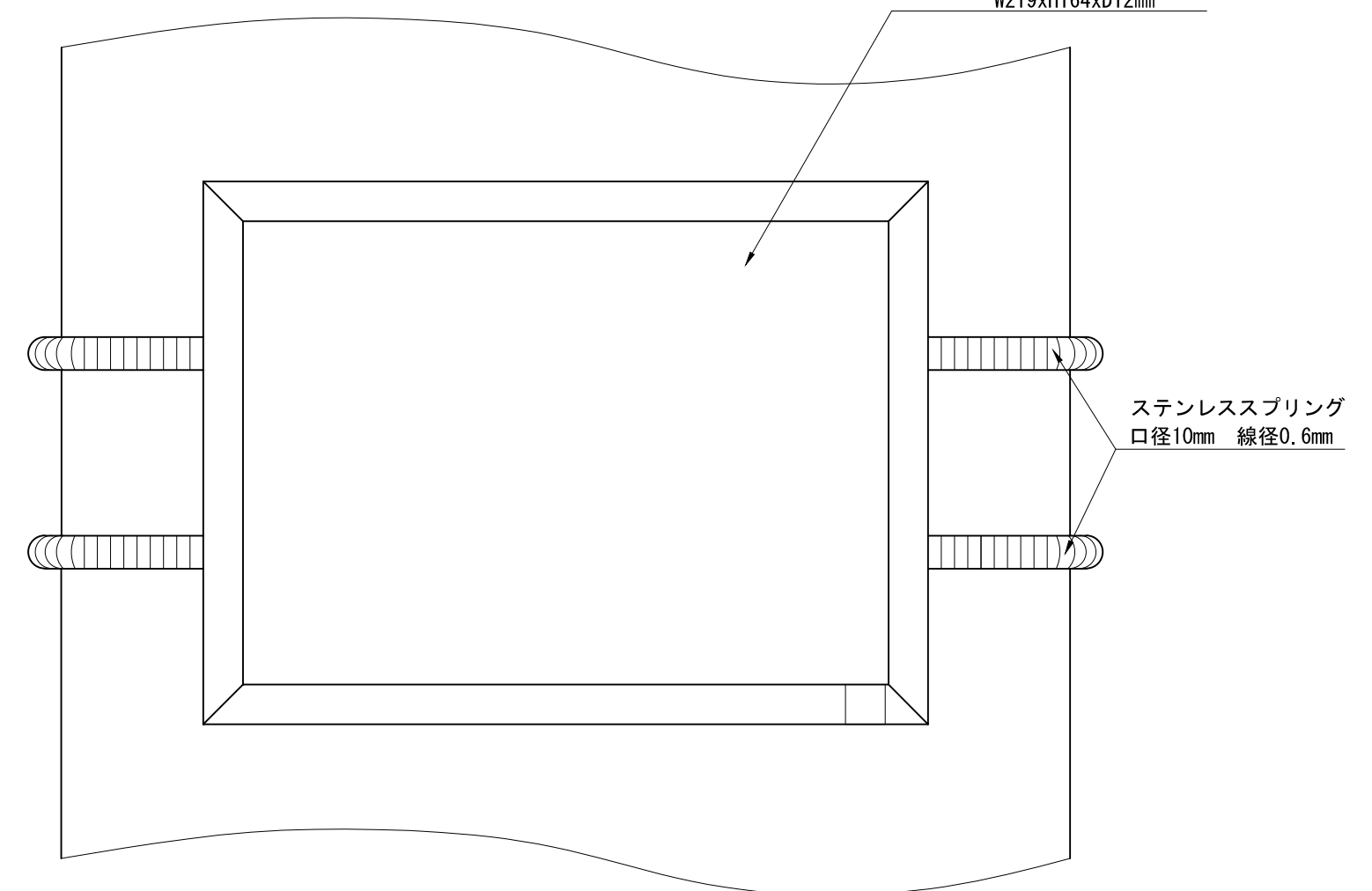
正面図 S=1:2
