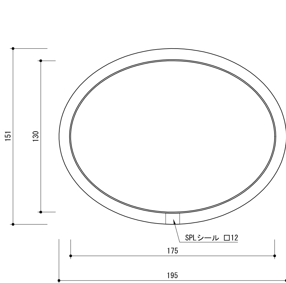
正面図 S=1:2
